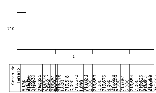
Estaca: 936+6,309 Cota do terreno: 713,573
