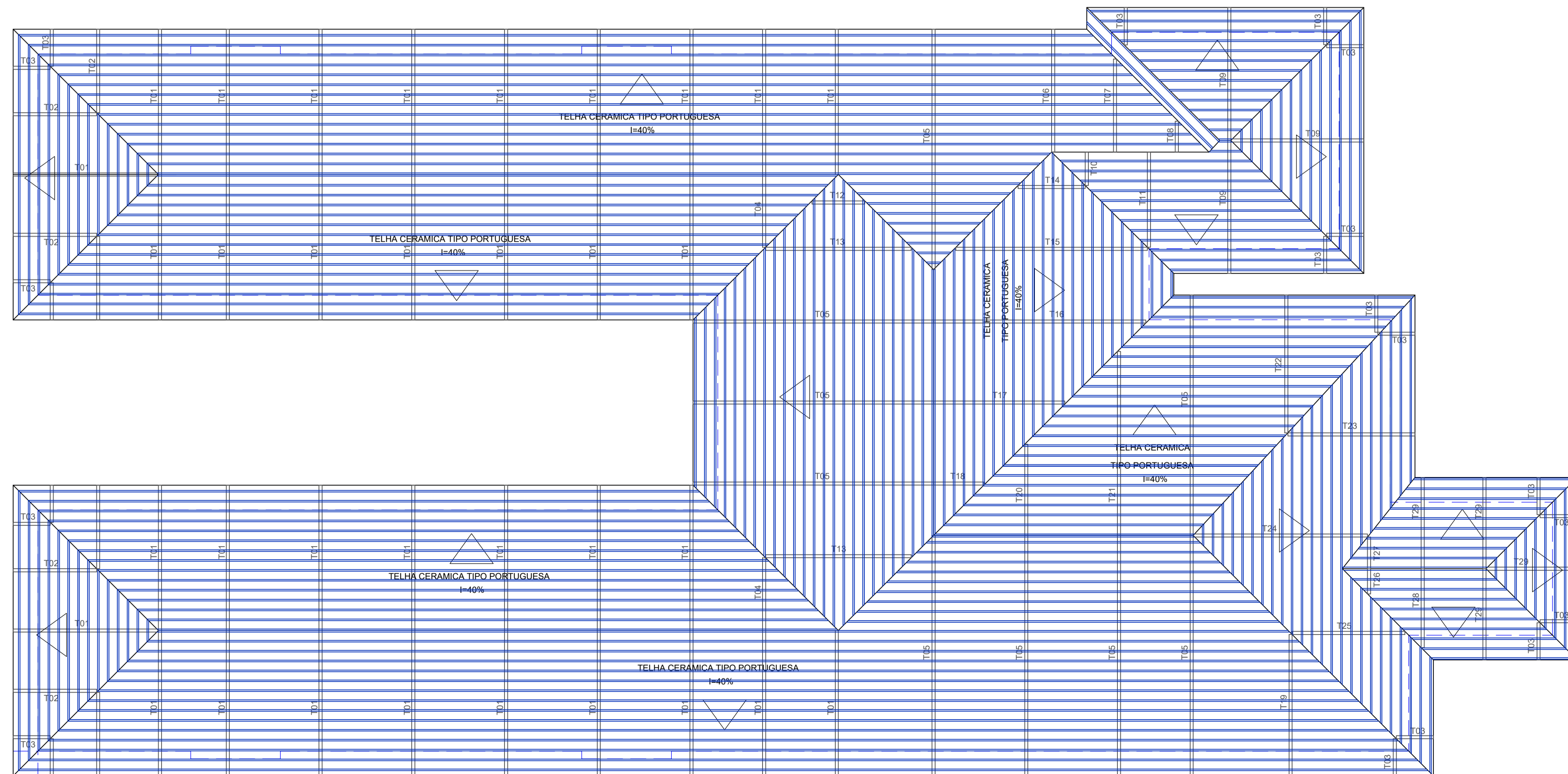
Planta de Cobertura - Detalhes Tesouras Esc: 1/100
