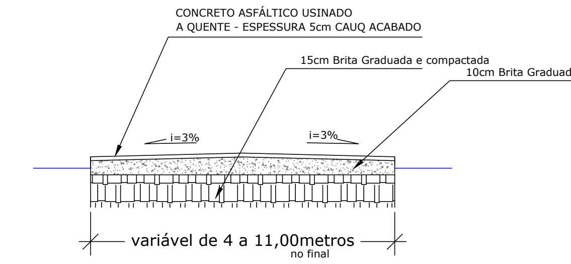
CORTE ESQUEMÁTICO - RUA ESCALA 1/25
