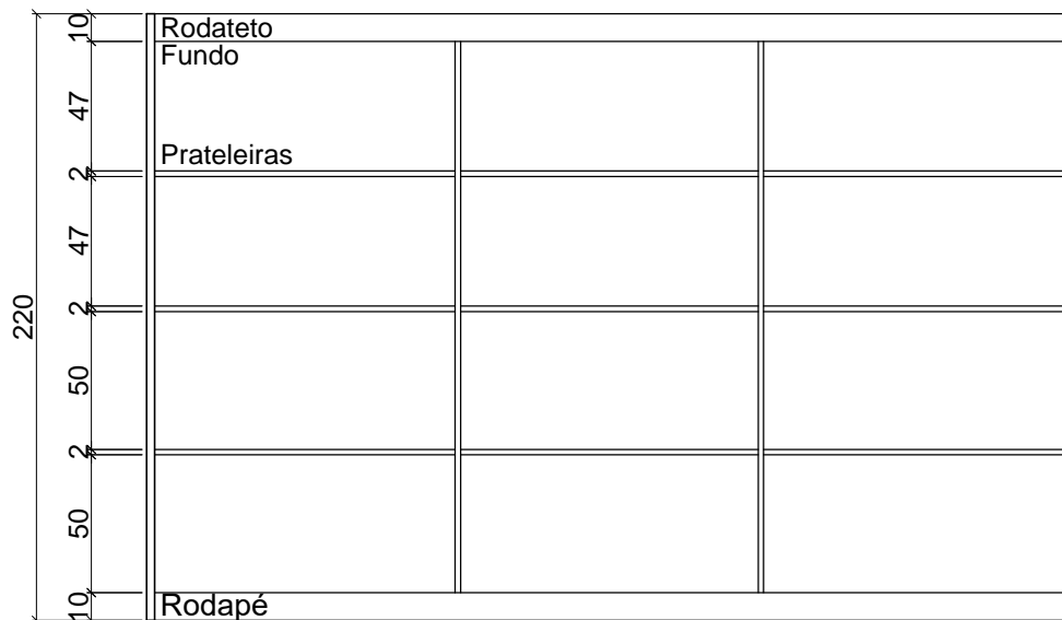
VISTA FRONTAL INTERNA - ARMÁRIO 01
