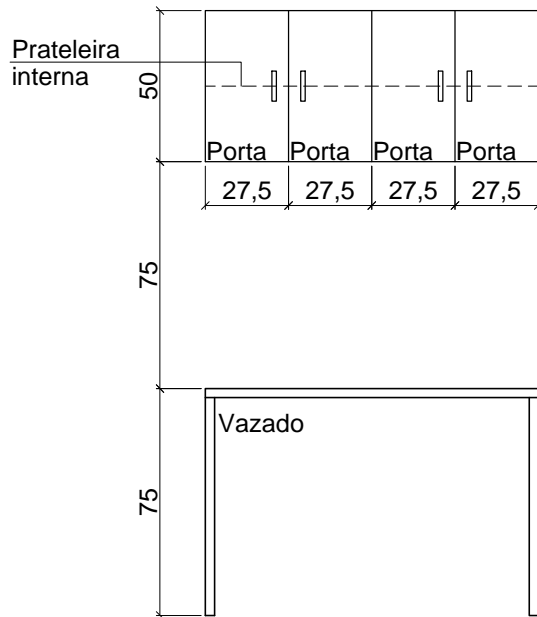
VISTA FRONTAL ESC _____ 1:25
