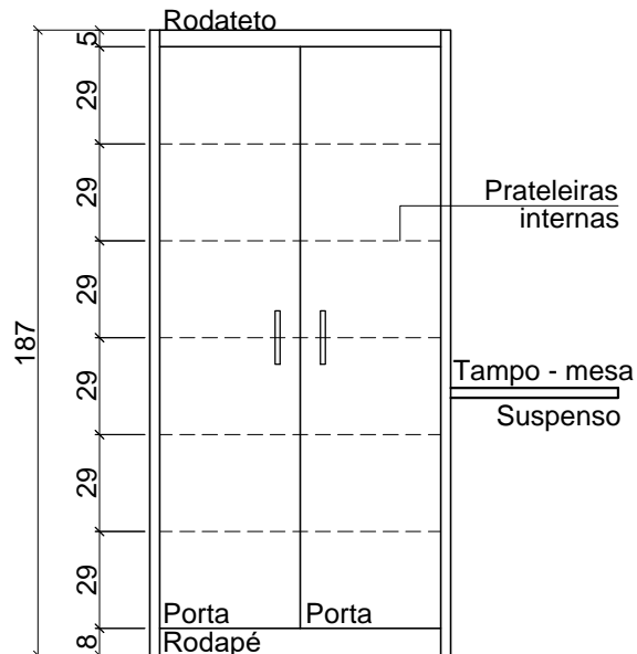
VISTA FRONTAL - ARMÁRIO ESC. 1:25
