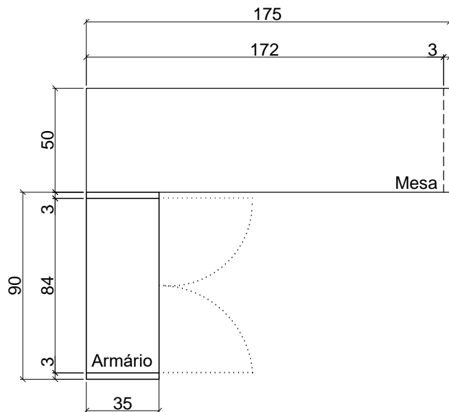
VISTA SUPERIOR ESC. 1:25
