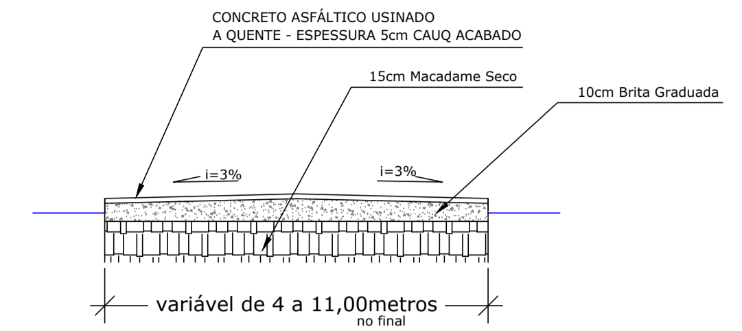
CORTE ESQUEMÁTICO - RUA ESCALA 1/25
