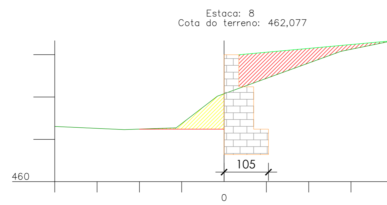
PERFIL MURO - LATERAL SUBIDA DIREITA ESCALA 1/50
