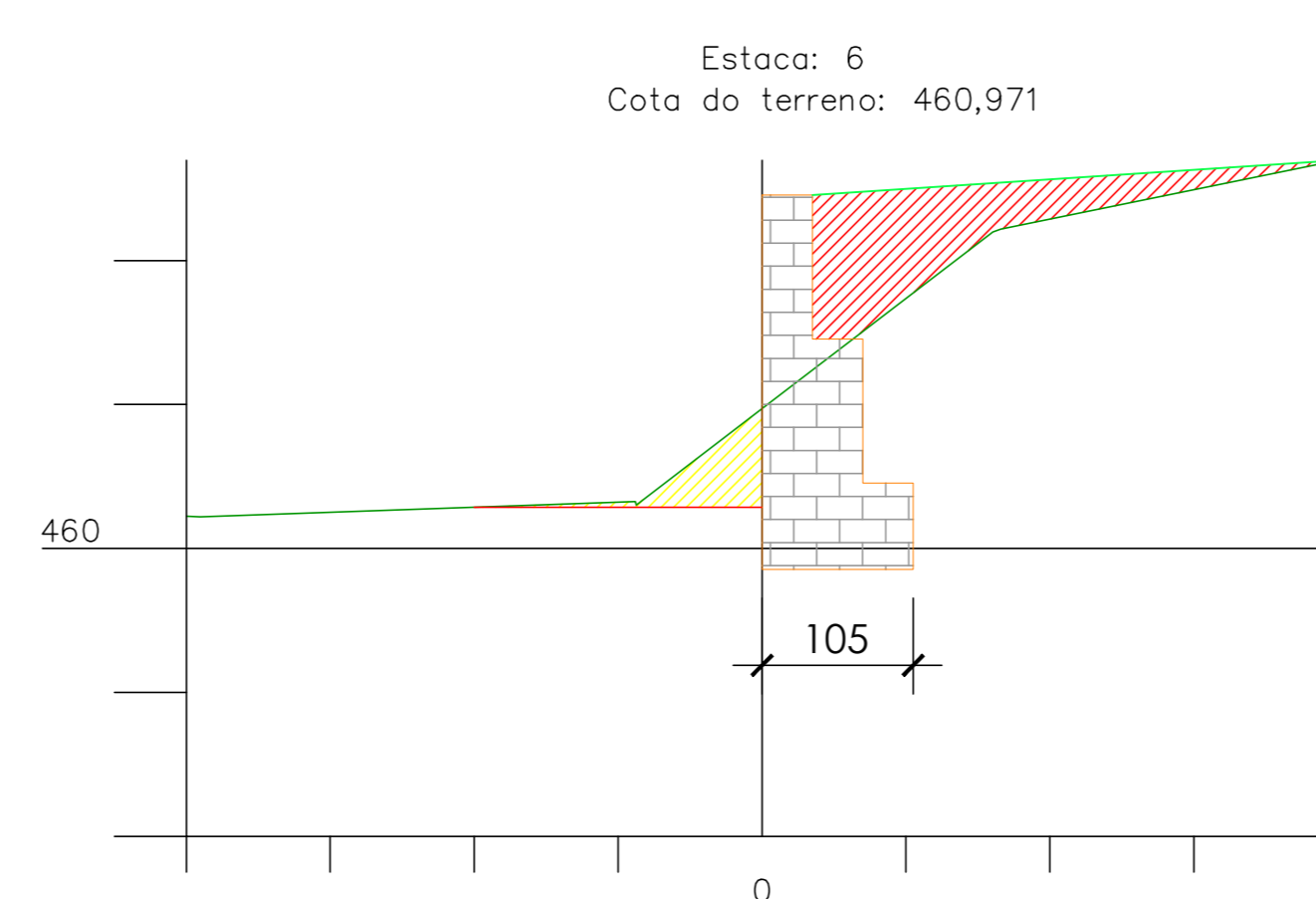
DETALHES SEÇÕES MURO - LATERAL SUBIDA DIREITA ESCALA 1/50
