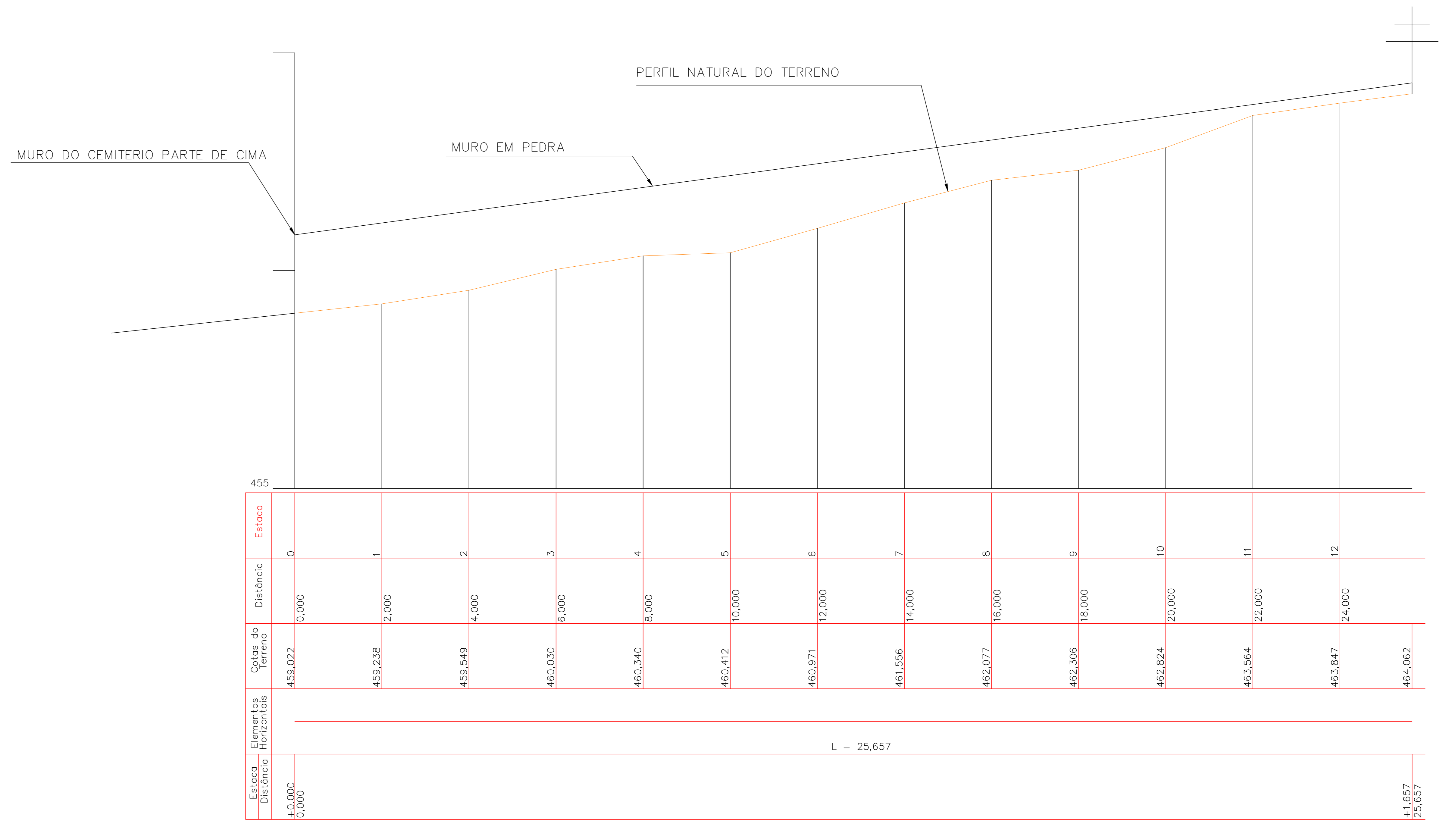
PERFIL MURO - LATERAL SUBIDA DIREITA ESCALA 1/50
