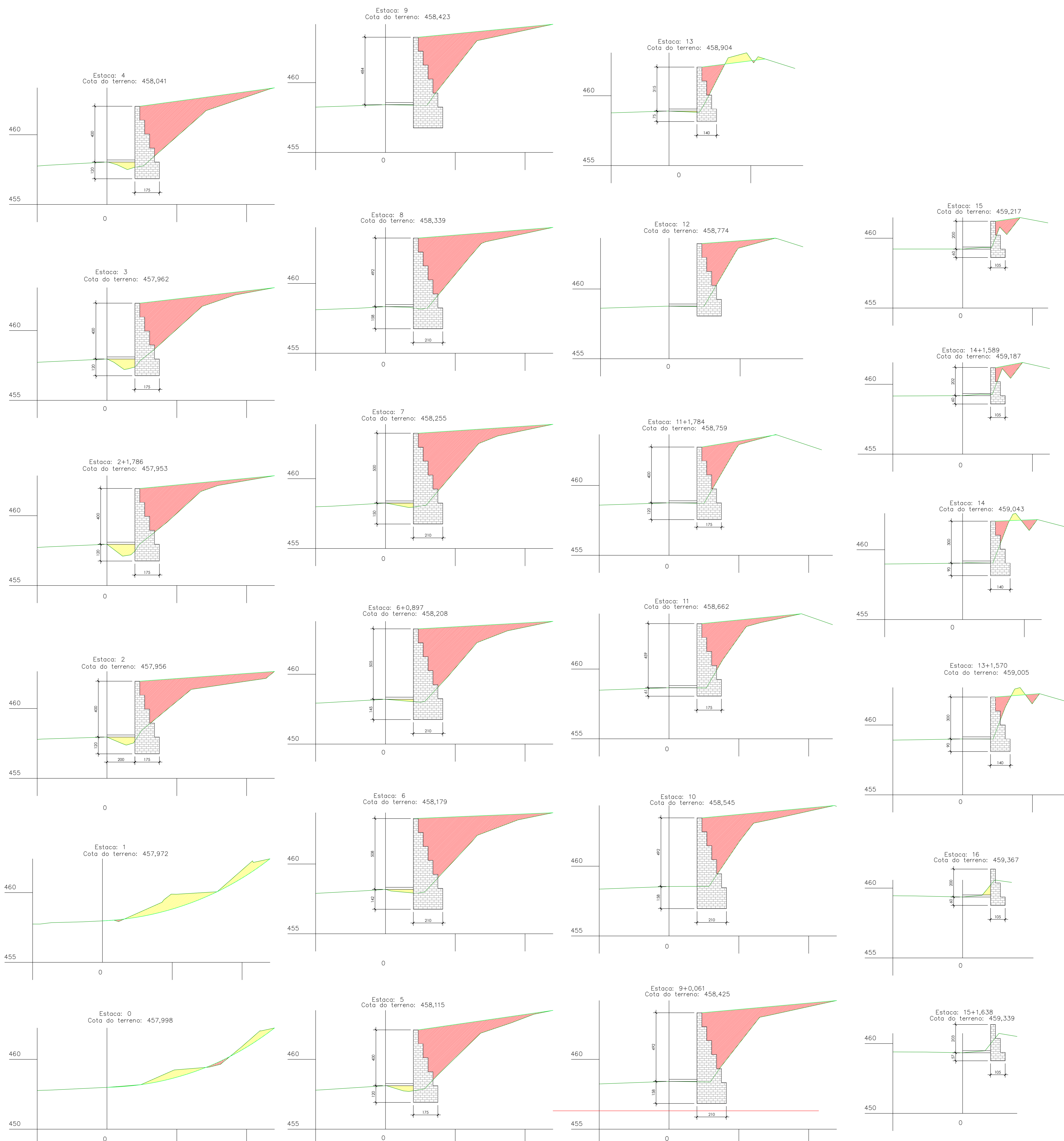
DETALHES SEÇÕES MURO FRONTAL ESCALA 1/50
